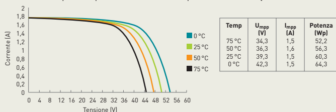
Curve di potenza per diversi valori di temperatura Modulo tipo SCG60-HV-F
